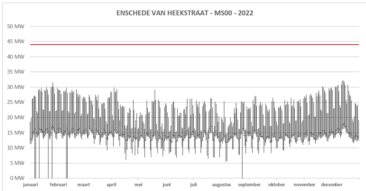
Figuur 2. Gemeten transportbelasting op HS/MS-station Enschede Van Heekstraat MS00 in 2022. Een positieve waarde representeert afname van het hoogspanningsnet. De aanwezige transportcapaciteit voor afname bedraagt 44,0 MW.
