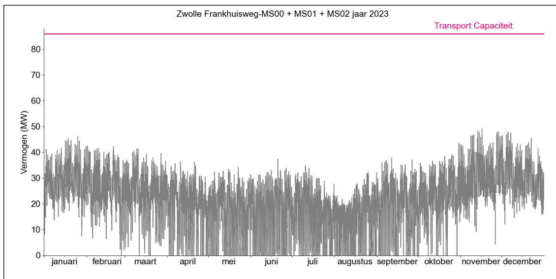
Figuur 2. Gerealiseerde transportbelasting voor afname op HS/MS-station Zwolle Frankhuisweg MS00 + MS01 + MS02 in 2023.
