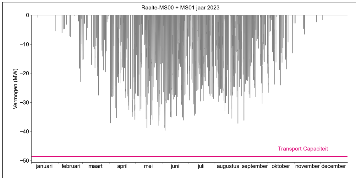
Figuur 2. Gerealiseerde transportbelasting voor invoeding op HS/MS-station Raalte MS00 + MS01 in 2023.
