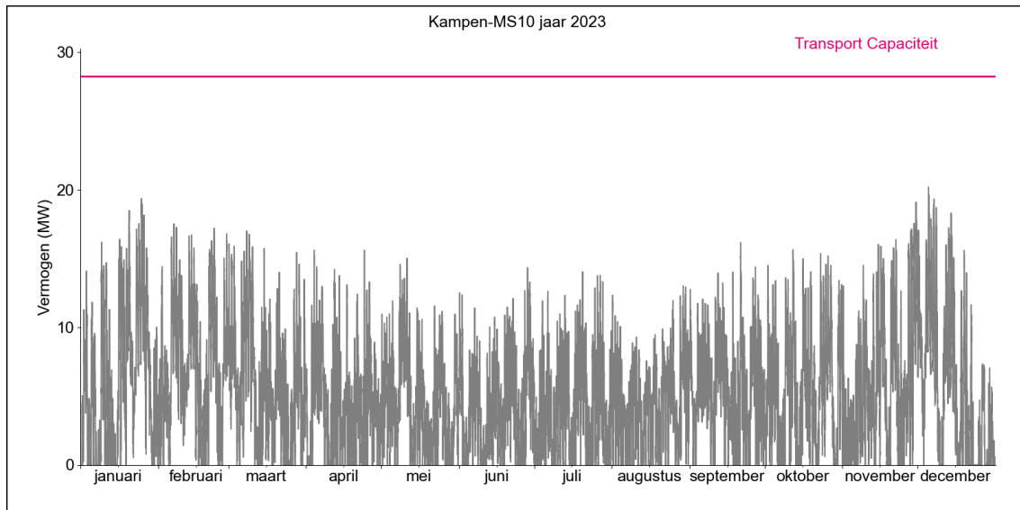
Figuur 2. Gerealiseerde transportbelasting voor afname op HS/MS-station Kampen MS10 in 2023.
