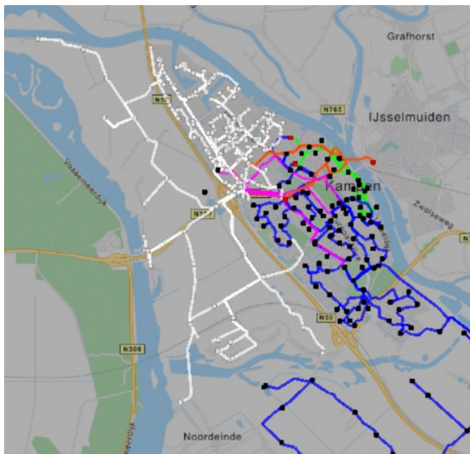
Figuur 1. Geografische indicatie van het voorzieningsgebied van HS/MS-station Kampen MS10 (in wit).
