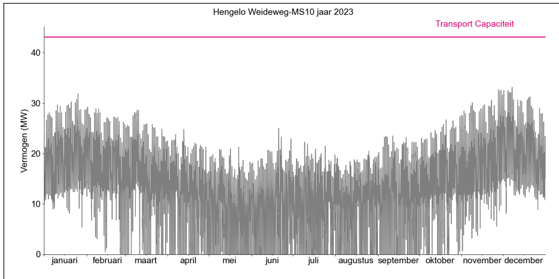
Figuur 2. Gerealiseerde transportbelasting voor afname op HS/MS-station Hengelo Weideweg MS10 in 2023.
