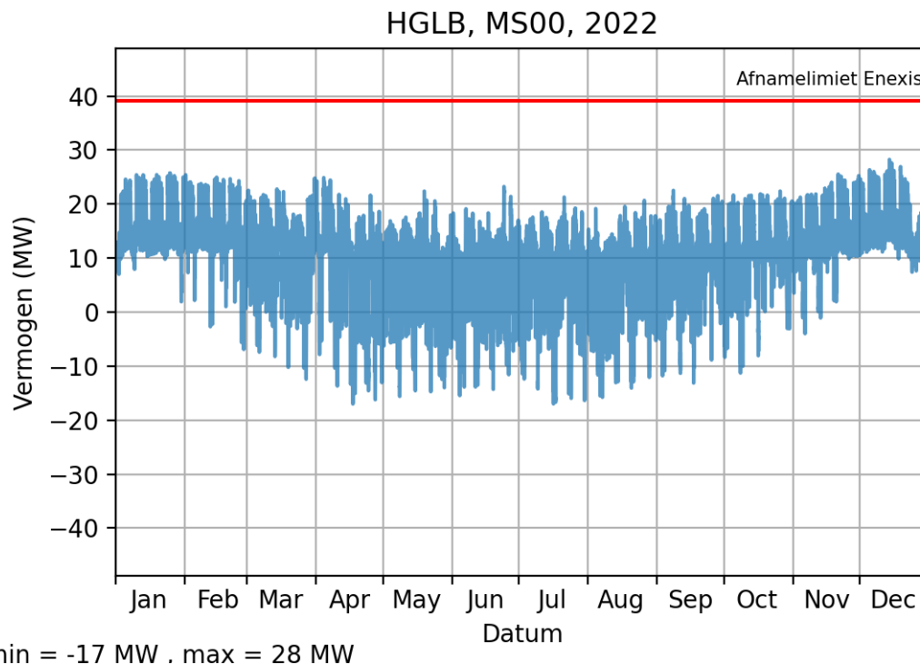
Figuur 2. Gemeten transportbelasting op HS/MS-station Hengelo Boldershoek blok 00 in 2022. Een positieve waarde representeert afname van het hoogspanningsnet. De aanwezige transportcapaciteit voor afname bedraagt 39,1 MW.
