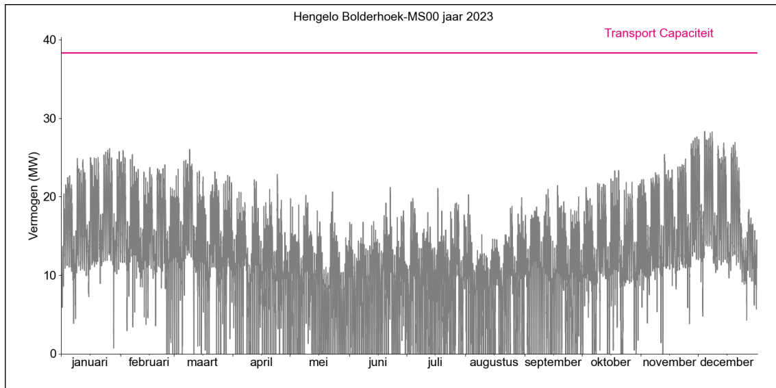
Figuur 2. Gerealiseerde transportbelasting voor afname op HS/MS-station Hengelo Bolderhoek MS00 in 2023.
