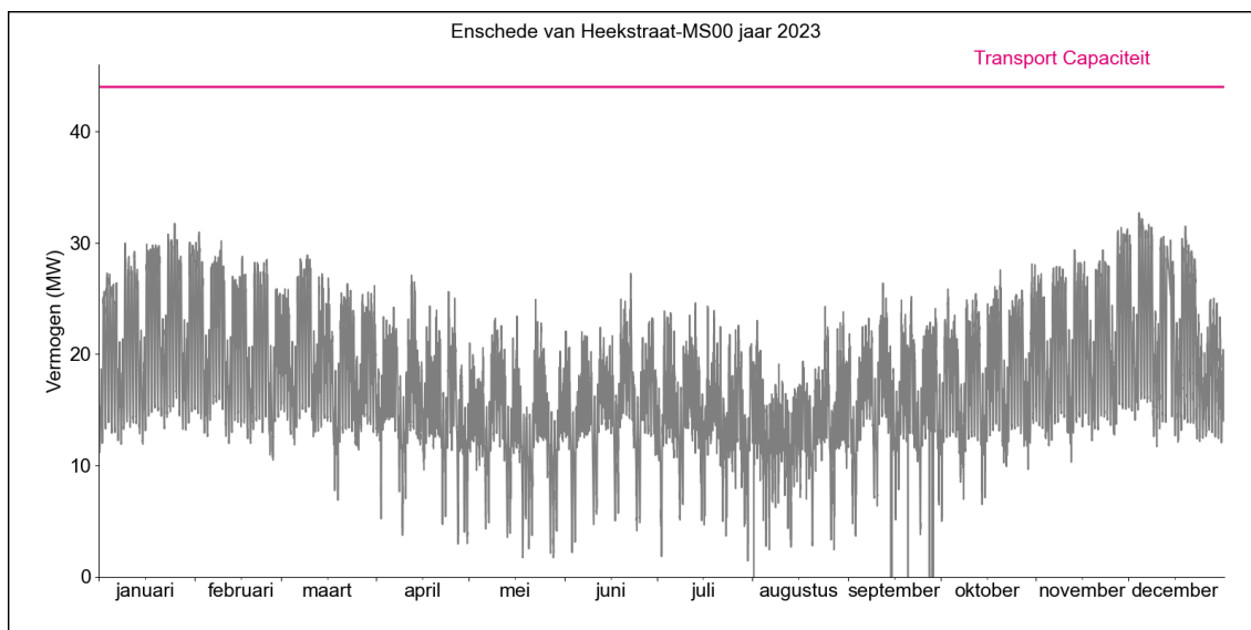
Figuur 2. Gerealiseerde transportbelasting voor afname op HS/MS-station Enschede van Heekstraat MS00 in 2023.
