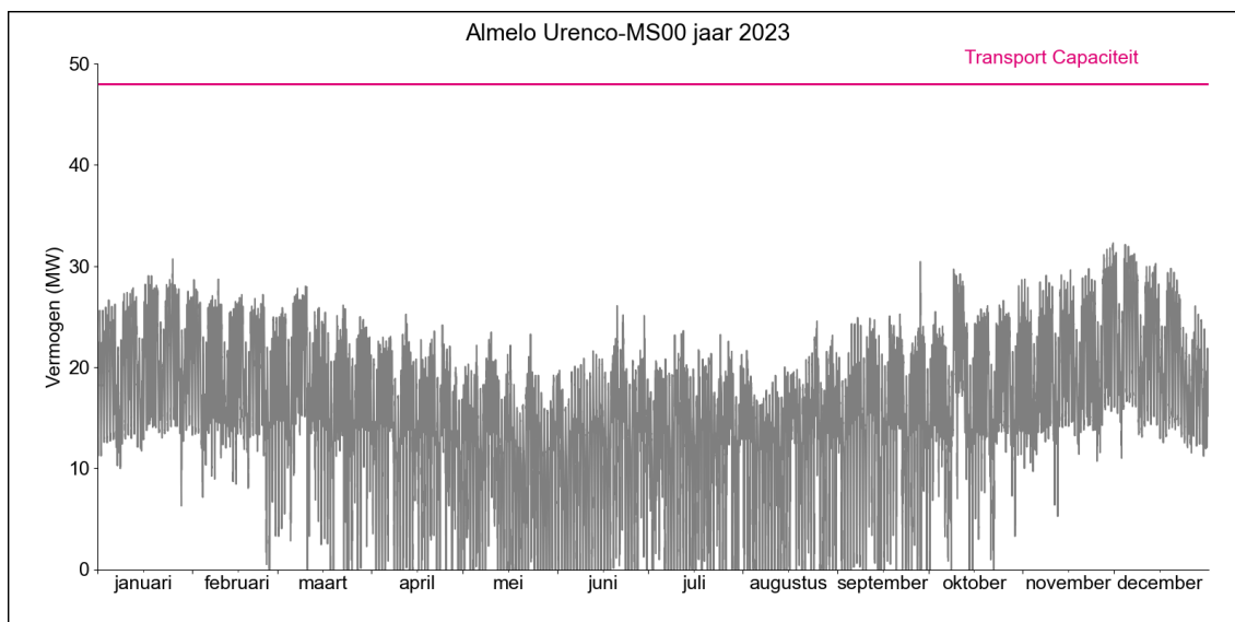
Figuur 2. Gerealiseerde transportbelasting voor afname op HS/MS-station Almelo Urenco MS00 in 2023.
