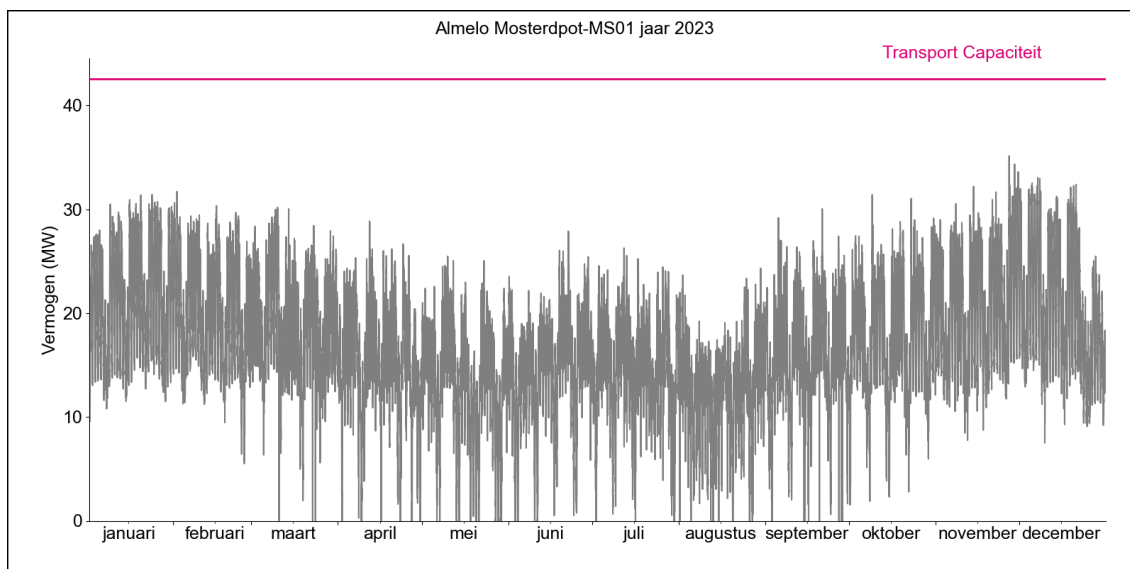
Figuur 1. Gerealiseerde transportbelasting voor afname op HS/MS-station Almelo Mosterdpot MS01 in 2023.
