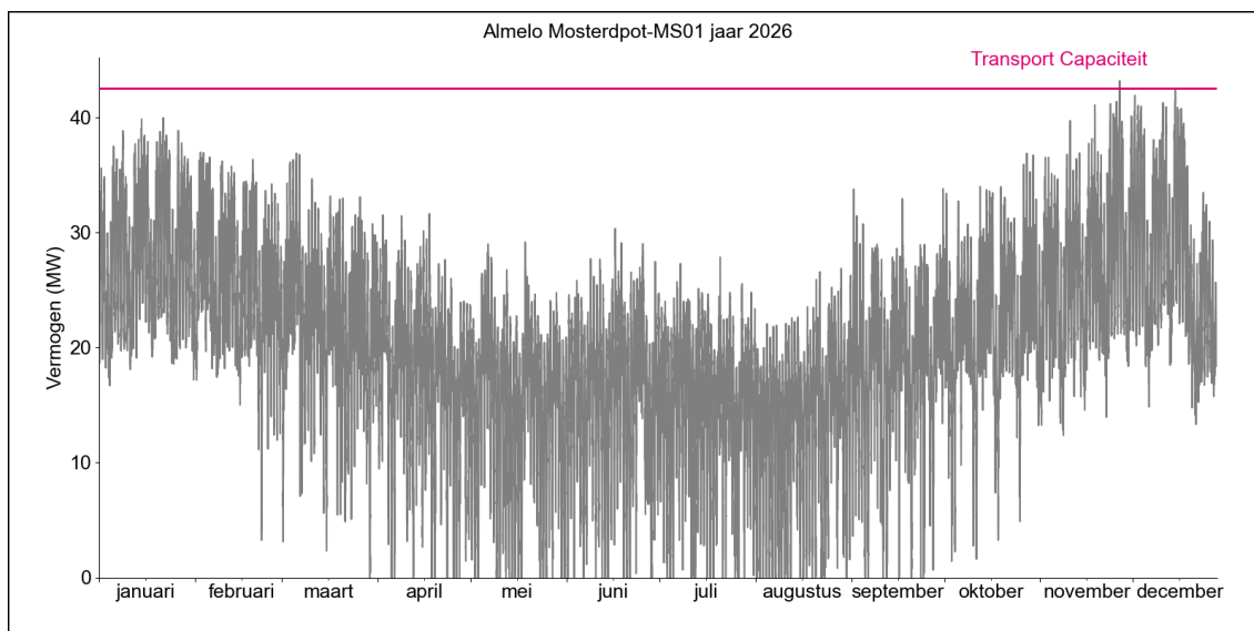
Figuur 2. Prognose van de benodigde transportcapaciteit in 2026.
