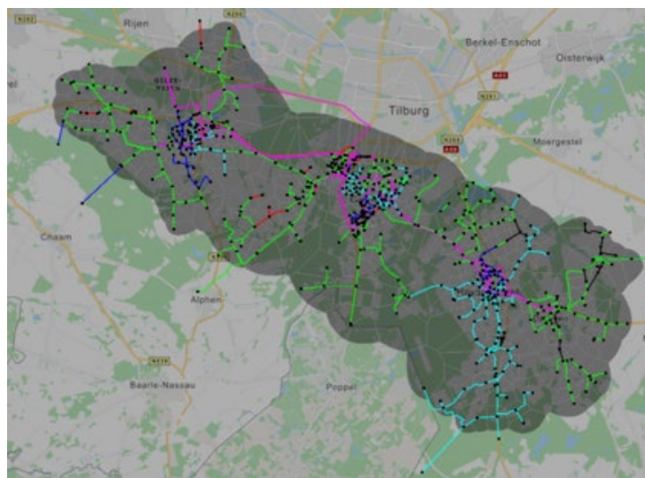
Figuur 1. Geografische indicatie van het voorzieningsgebied van HS/MS-station Tilburg Zuid Blok B.
