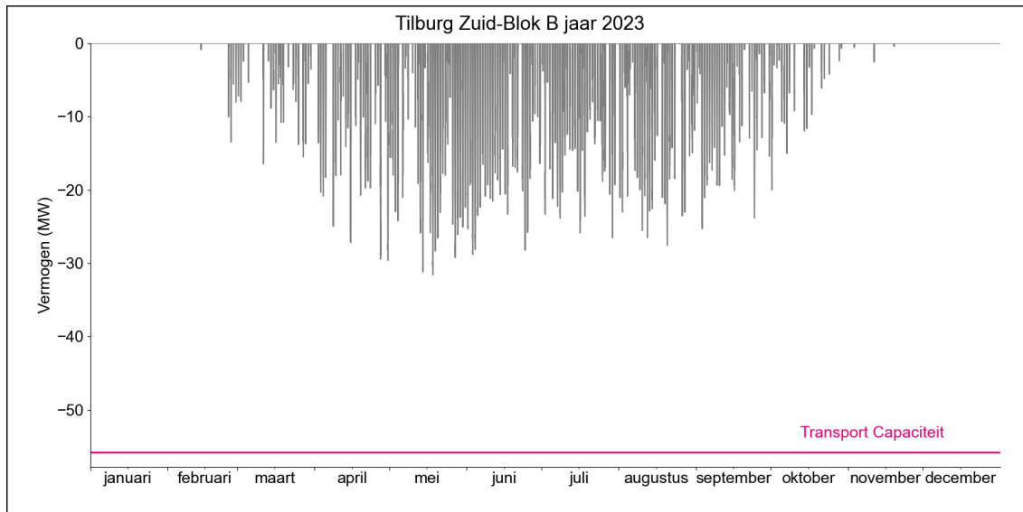
Figuur 2. Gerealiseerde transportbelasting voor invoeding op HS/MS-station Tilburg Zuid Blok B in 2023.
