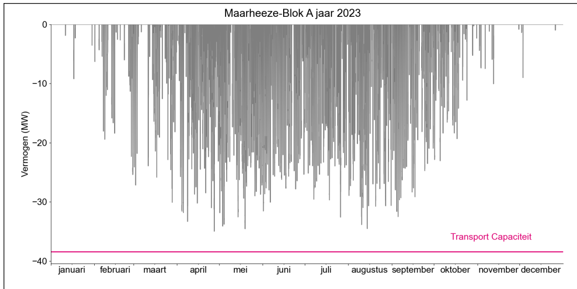
Figuur 2. Gerealiseerde transportbelasting voor invoeding op HS/MS-station Maarheeze Blok A in 2023.
