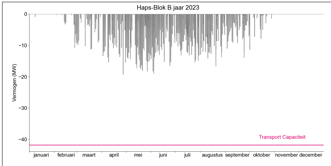
Figuur 2. Gerealiseerde transportbelasting voor invoeding op HS/MS-station Haps Blok B in 2023.
