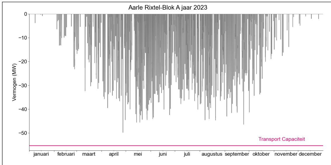
Figuur 2. Gerealiseerde transportbelasting voor invoeding op HS/MS-station Aarle-Rixtel Blok A in 2023.
