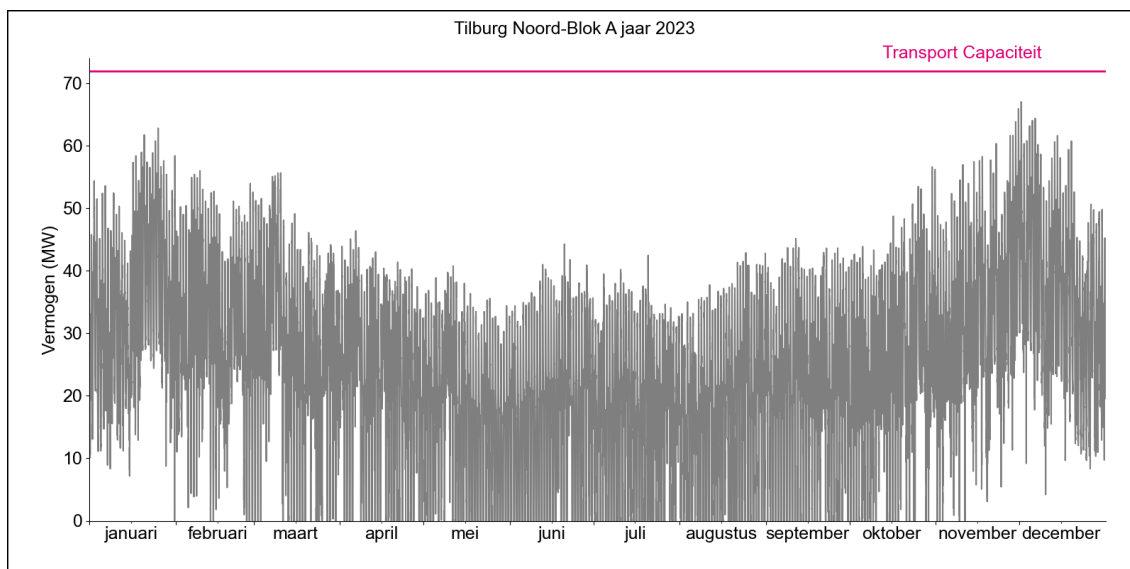
Figuur 2. Gerealiseerde transportbelasting voor afname op HS/MS-station Tilburg Noord Blok A in 2023.
