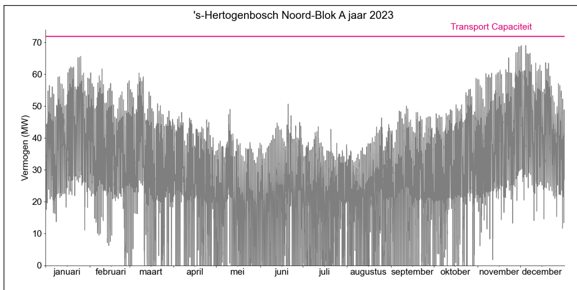
Figuur 2. Gerealiseerde transportbelasting voor afname op HS/MS-station 's-Hertogenbosch Noord Blok A in 2023.
