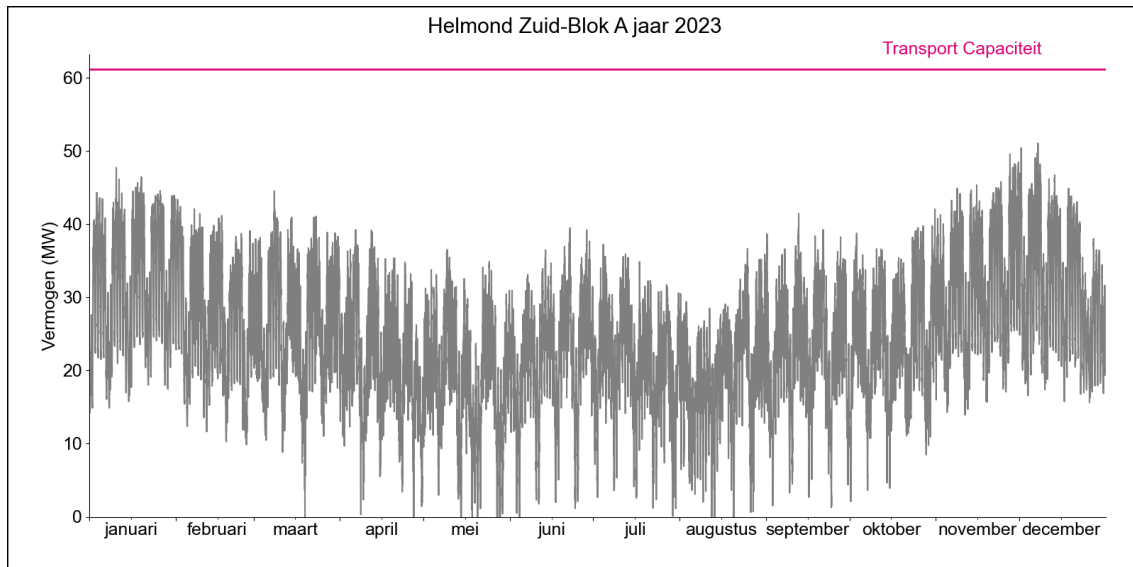
Figuur 2. Gerealiseerde transportbelasting voor afname op HS/MS-station Helmond Zuid Blok A in 2023.
