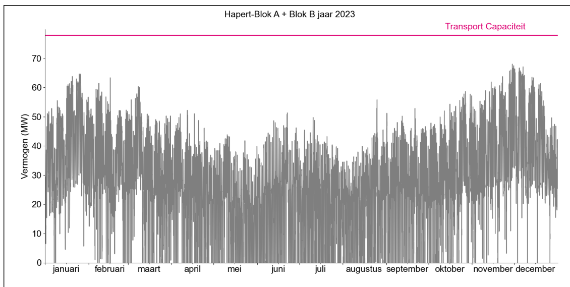
Figuur 2. Gerealiseerde transportbelasting voor afname op HS/MS-station Hapert Blok A + Blok B in 2023.
