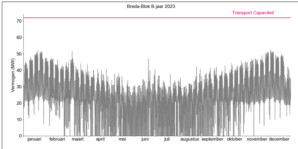
Figuur 2. Gerealiseerde transportbelasting voor afname op HS/MS-station Breda Blok B in 2023.
