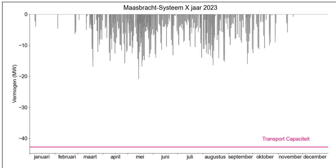
Figuur 2. Gerealiseerde transportbelasting voor invoeding op HS/MS-station Maasbracht Systeem X in 2023.
