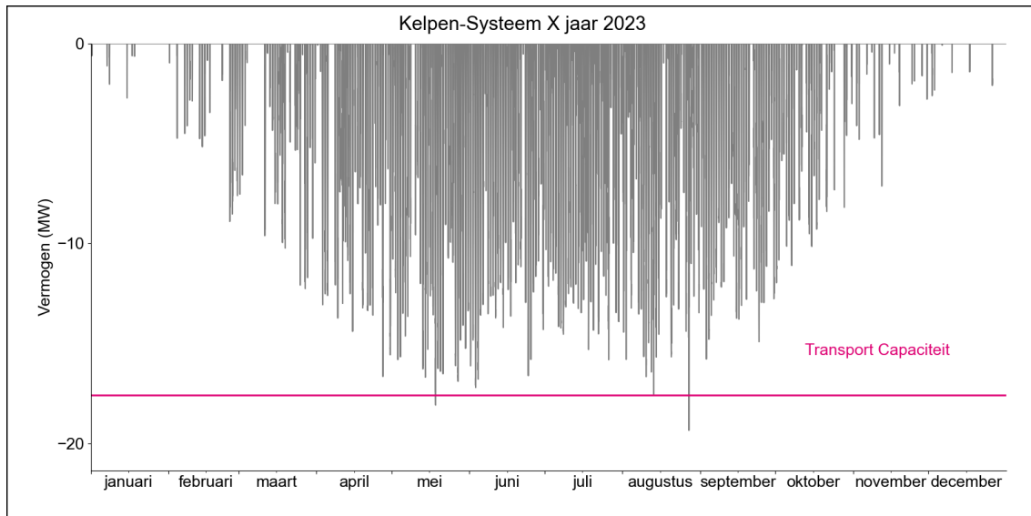
Figuur 2. Gerealiseerde transportbelasting voor invoeding op HS/MS-station Kelpen Systeem X in 2023.
