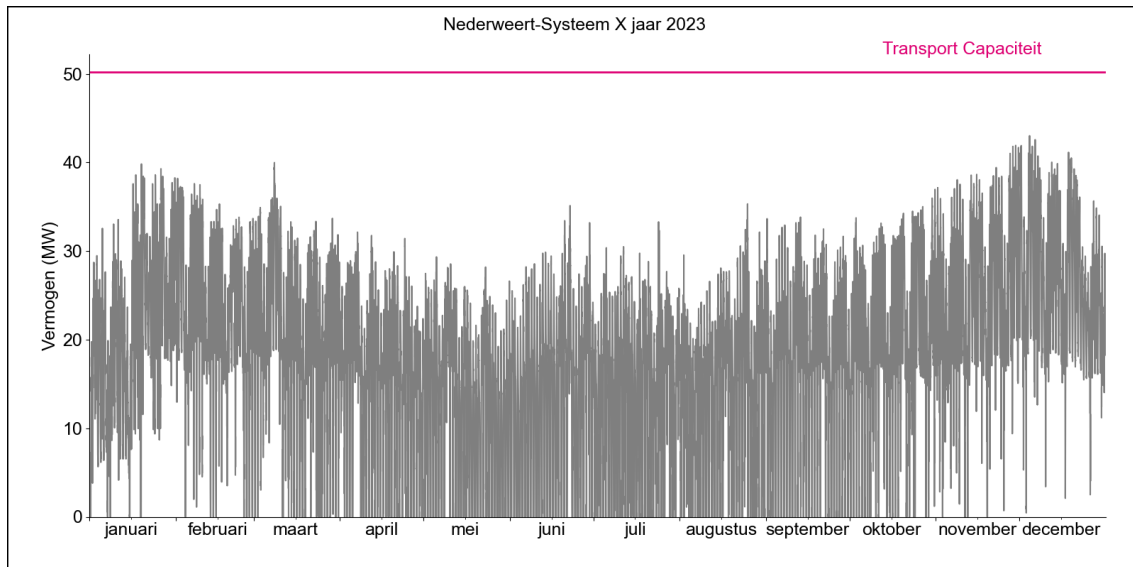
Figuur 2. Gerealiseerde transportbelasting voor afname op HS/MS-station Nederweert Systeem X in 2023.
