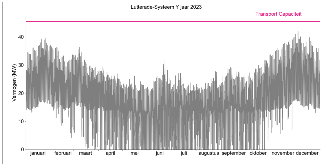
Figuur 2. Gerealiseerde transportbelasting voor afname op HS/MS-station Lutterade Systeem Y in 2023.
