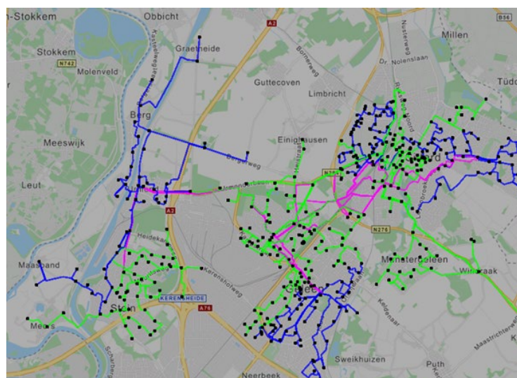
Figuur 1. Geografische indicatie van het voorzieningsgebied van HS/MS-station Lutterade Systeem Y.
