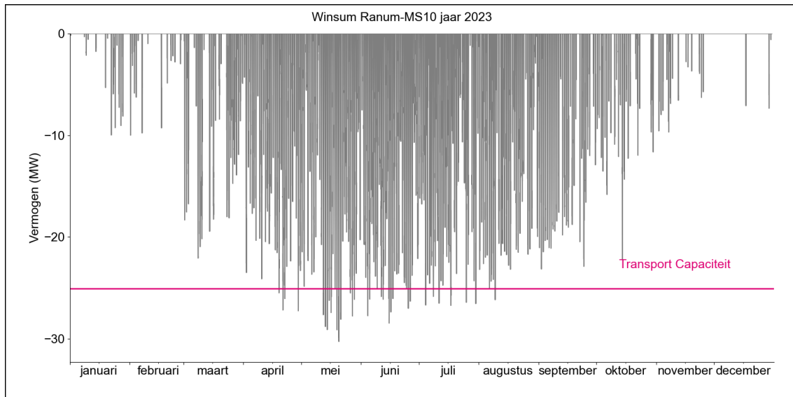
Figuur 2. Gerealiseerde transportbelasting voor invoeding op HS/MS-station Winsum Ranum MS10 in 2023.
