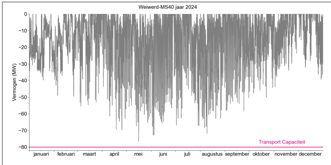
Figuur 2. Gerealiseerde transportbelasting voor invoeding op HS/MS-station Weiwerd MS40 in 2024.
