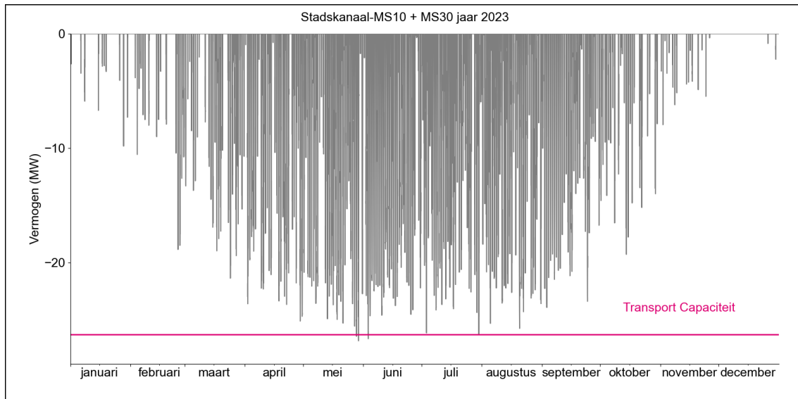
Figuur 2. Gerealiseerde transportbelasting voor invoeding op HS/MS-station Stadskanaal MS10 + MS30 in 2023.
