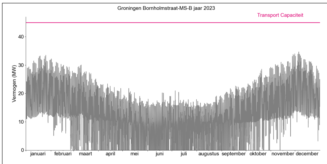
Figuur 2. Gerealiseerde transportbelasting voor afname op HS/MS-station Groningen Bornholmstraat MS-B in 2023.
