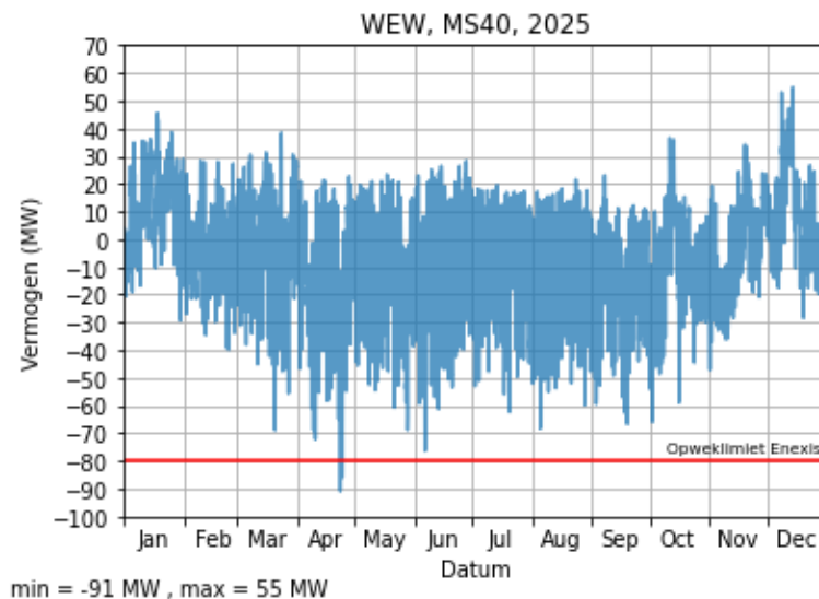
Figuur 3. Verwachte transportbelasting op station Weiwerd blok 40 in het laatste jaar van de congestie.
