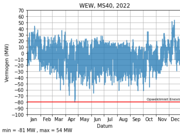
Figuur 2. Gemeten transportbelasting op station Weiwerd blok 40 in 2022. Een negatieve waarde representeert invoeding in het hoogspanningsnet. De huidige, aanwezige transportcapaciteit voor invoeding bedraagt 80 MW.
