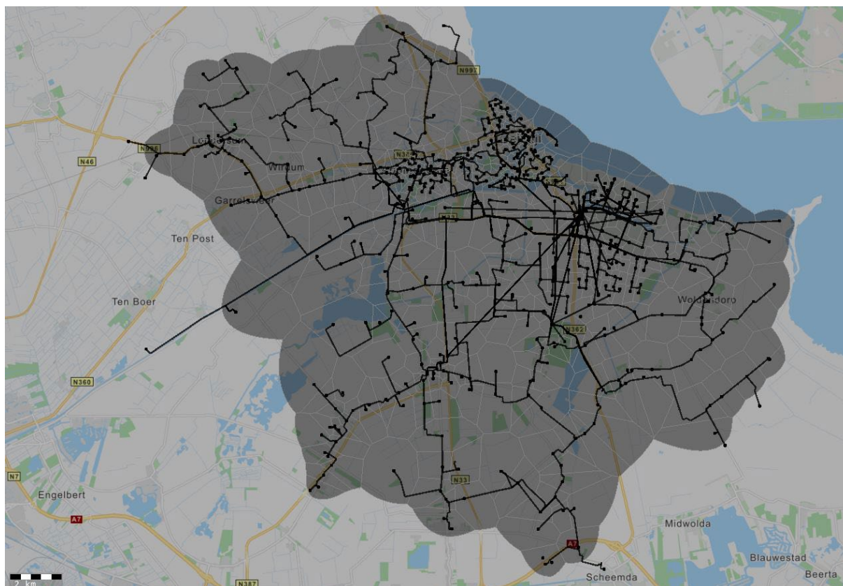
Figuur 1. Geografische indicatie van het voorzieningsgebied van HS/MS station Weiwerd blok 40.
