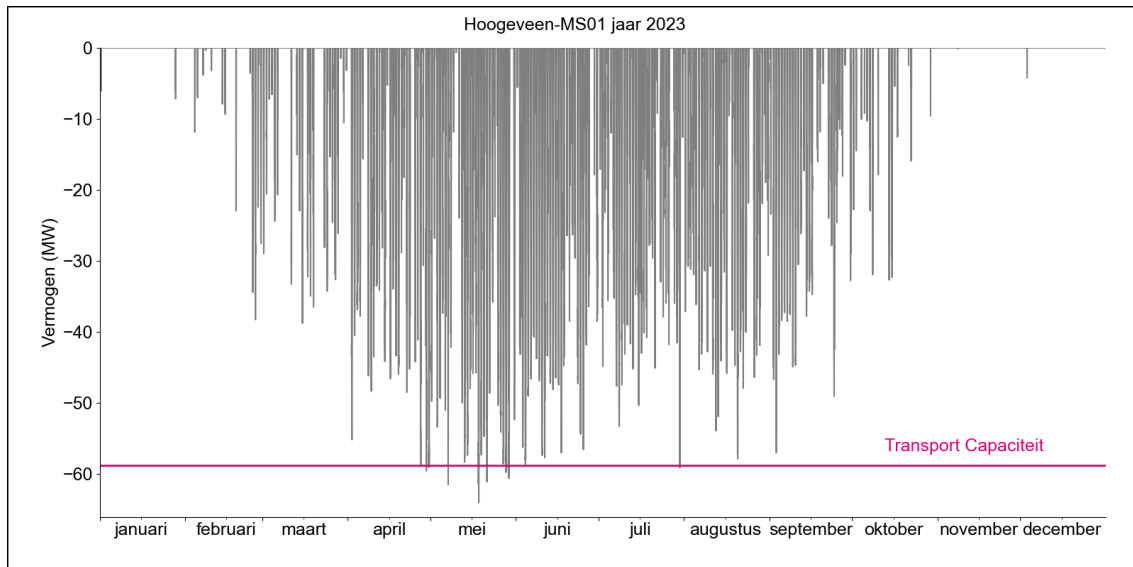
Figuur 2. Gerealiseerde transportbelasting voor invoeding op HS/MS-station Hoogeveen MS01 in 2023.
