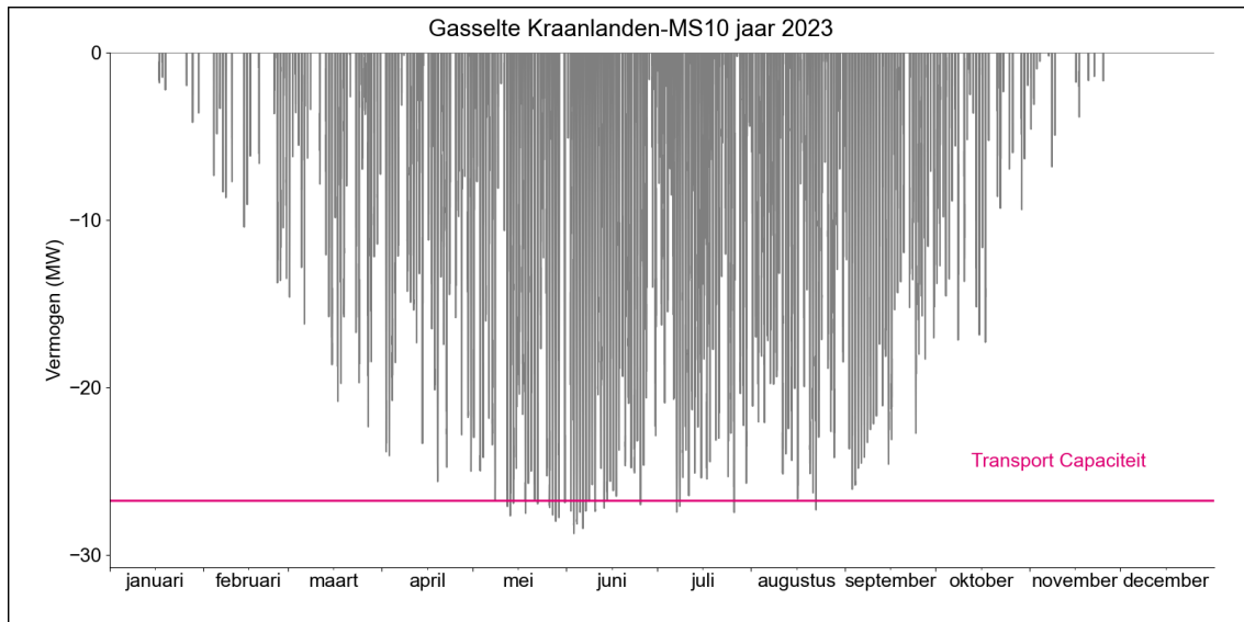
Figuur 2. Gerealiseerde transportbelasting voor invoeding op HS/MS-station Gasselte Kraanlanden MS10 in 2023.
