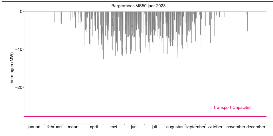
Figuur 2. Gerealiseerde transportbelasting voor invoeding op HS/MS-station Bargermeer MS50 in 2023.
