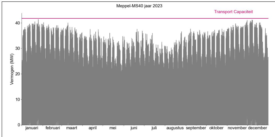
Figuur 2. Gerealiseerde transportbelasting voor afname op HS/MS-station Meppel MS40 in 2023.
