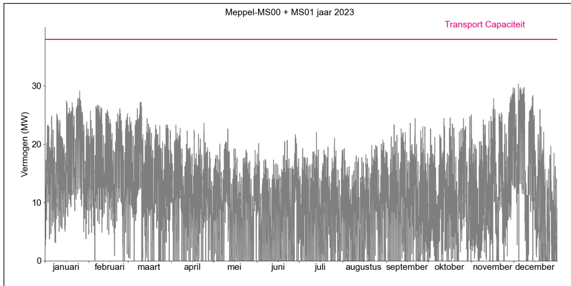
Figuur 2. Gerealiseerde transportbelasting voor afname op HS/MS-station Meppel MS00 + MS01 in 2023.
