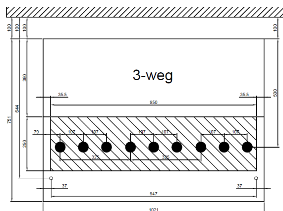
Afbeelding 6: vloerplan ABB Safeplus CCF
